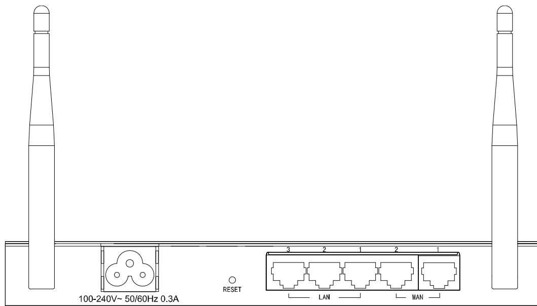
图 2-3 TL-WVR300后面板示意图
